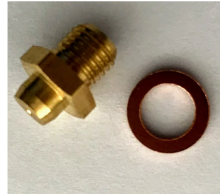
41261580 Одна форсунка сжиженный газ d.0,82 mm
